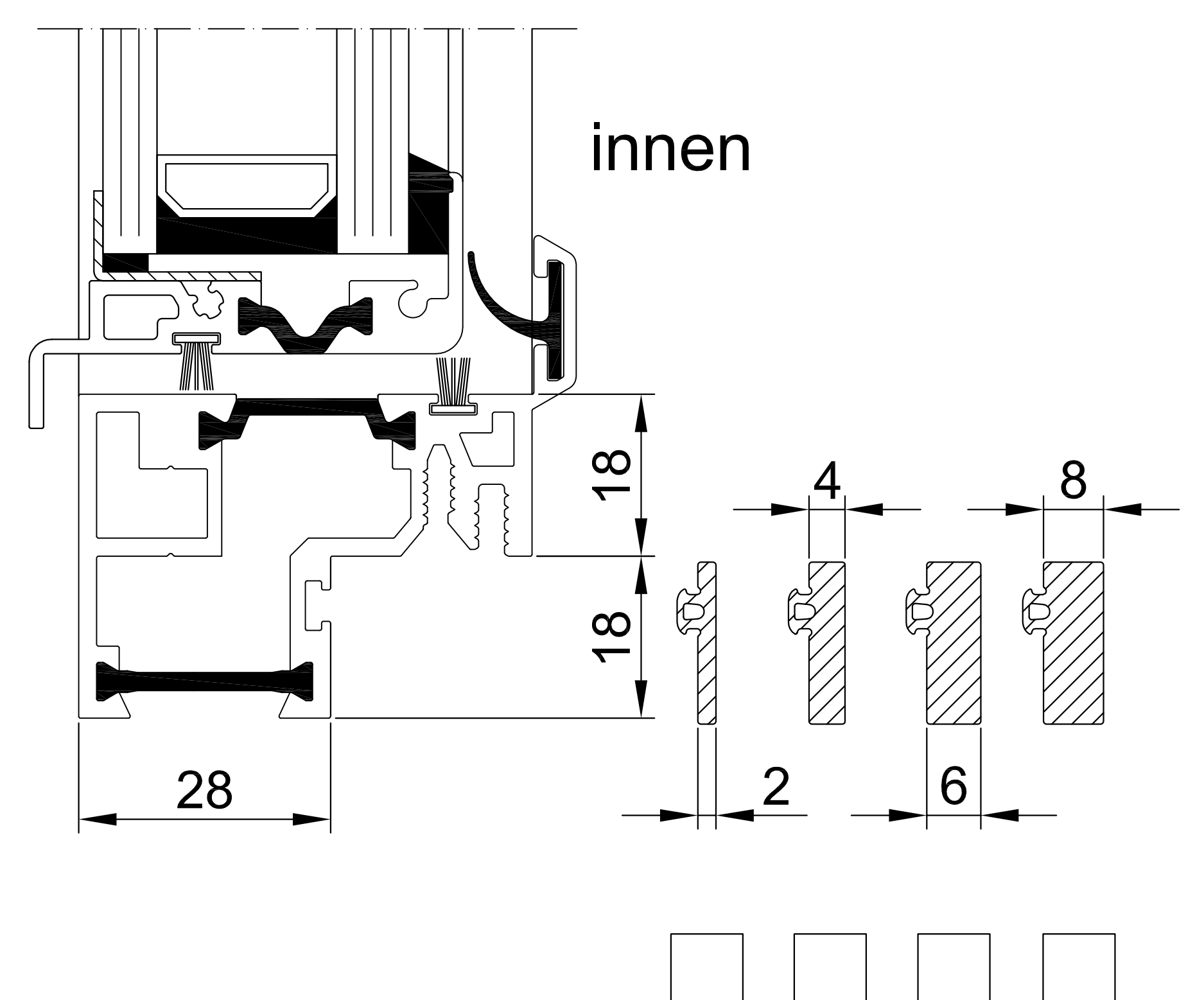
Detail Rahmen Typ 2
