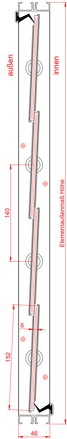
Detail Klemmrahmen Rahmen Typ 2
