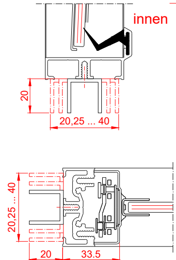
Detail Klemmrahmen Rahmen Typ 2
