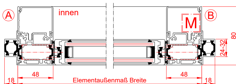
Rahmen Typ 2
