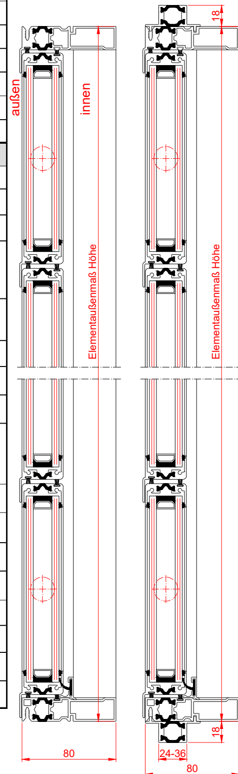
Rahmen Typ 1
