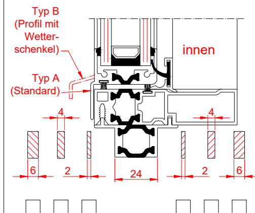
Detail Rahmen
