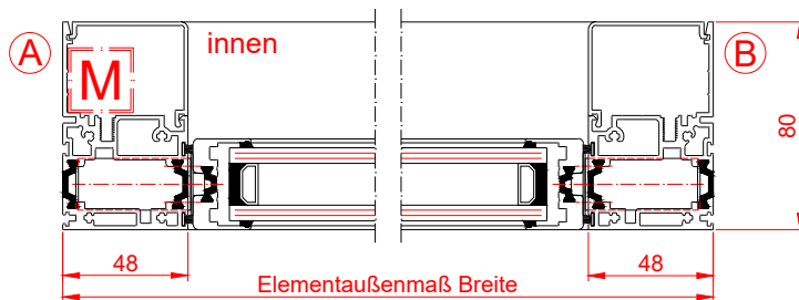
Rahmen Typ 1
